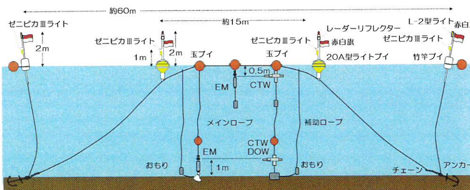
図-2 設置物の構造
