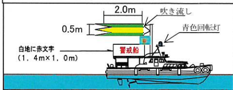
図6 警戒船
