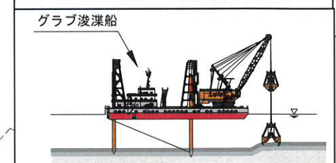
図3 浚渫船
