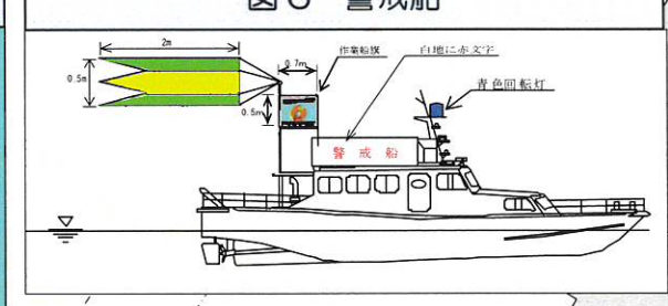
図6 警戒船
