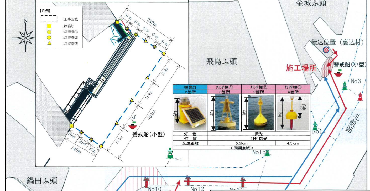
図3 施工状況：裏込工（ガット船）
