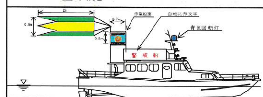
図7 警戒船
