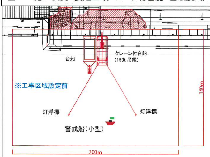
図4 施工状況：裏込工（クレーン付台船・自取投入）
