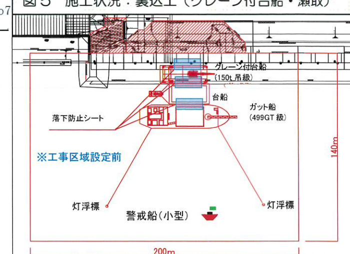
図5 施工状況：裏込工（クレーン付台船・瀨取）
