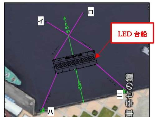
図2 係留姿図
