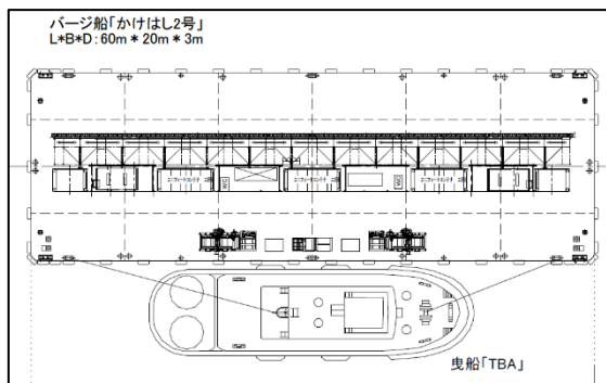
図5 赤レンガ入出航時 曳航図
