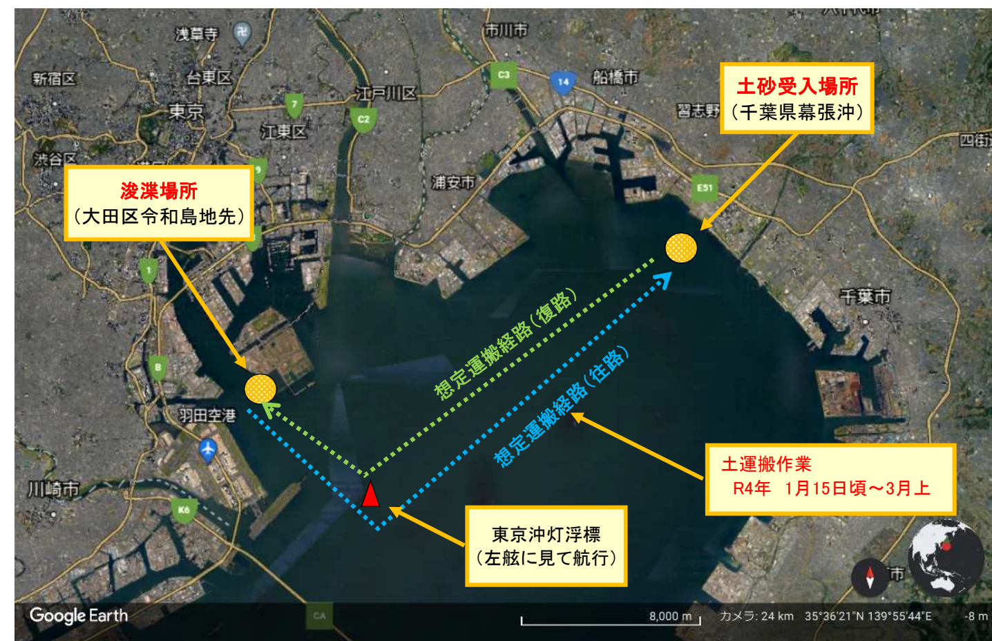
【施工位置図(潜水探査・浚渫)】
