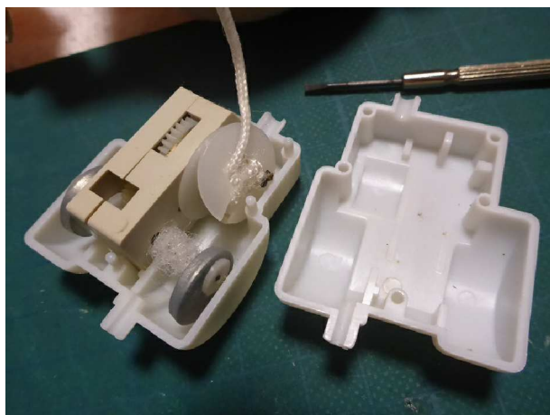
袋の中の構造部を開くと、繊維状の詰め物の絡みを発見し、除去する。丸く見えるのは、ゼンマイを巻き上げるドラム。
