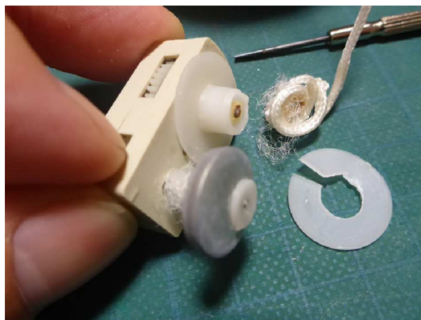
ドラム内にも繊維の絡みが入り込み、ドラムの片側のポリプロピレンが割れている。このままの接着は不可能。
