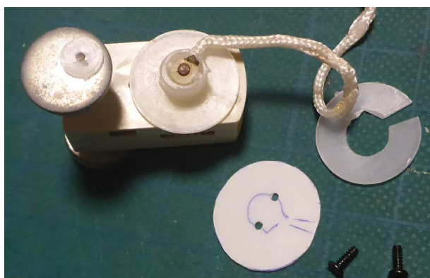
あらかじめ芯棒にヒモの端を固定した後、プラ板を円盤状に切り抜き。切り込みは不要。ビス2本で芯棒に固定。
