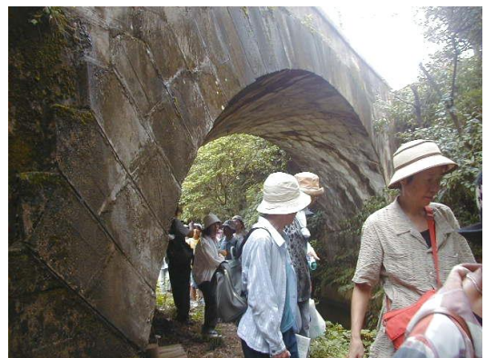
ねじり橋（六把野井水拱橋）
