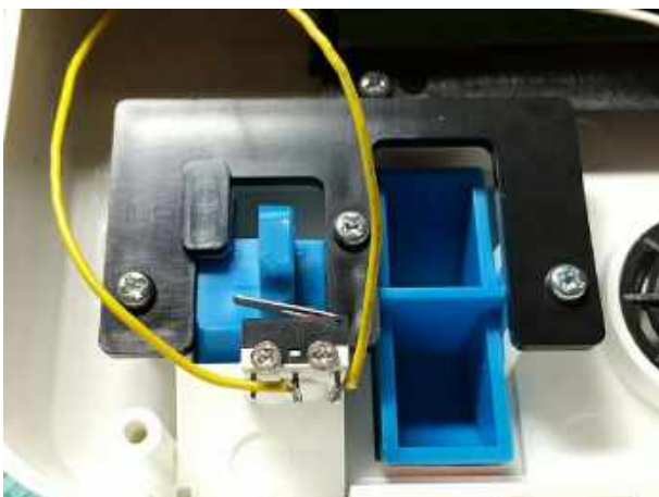
マイクロスイッチで代用、操作感は違うが、 レバー操作で走行音が出せるように改造
