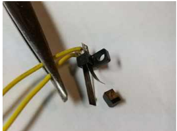
レバー操作の板状スイッチが変形し折損 在庫部品がなく、マイクロスイッチで代用
