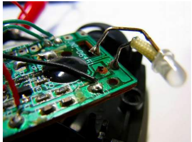
④ヘッドライト LEDが基板パターン剥離で断線 LEDを元位置に戻して再半田付けで固定する
