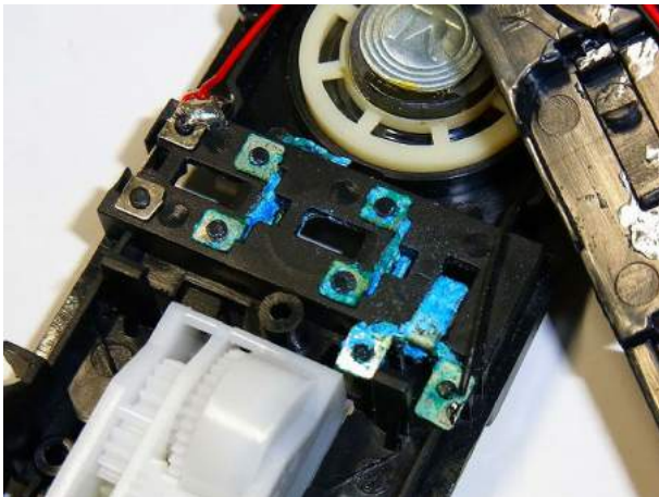
③電池BOXのウラ側までが電解液で真っ青 マイナス電極から配線の芯までも伝っていた
