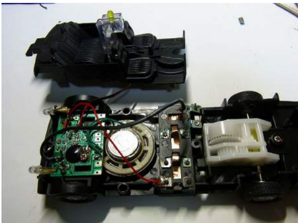
⑤りん青銅板でLR44の電池端子板を自作 マイナス側リード線を交換して応急処置完了
