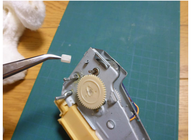
写真ではわかりにくいですが、ピニオンギヤがヒビ割れてモーター軸が空回りして、回転が次のギヤに伝達されていない状態。ここは強い力がかかるため接着補強では無理で、新品ギヤに交換する。
