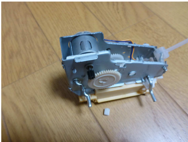
新しいギヤを取付けて動作確認。写真で黒く見えるのが交換後のピニオンギヤ。とりあえず動くように改善したので、今回の「治療」はここまで。外被覆の復元は大変苦労した。「キメ込み人形」の要領で完成。
