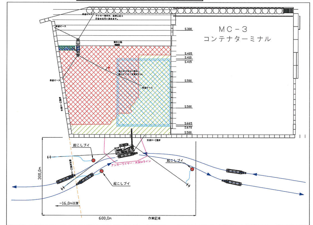
作業船配置図
