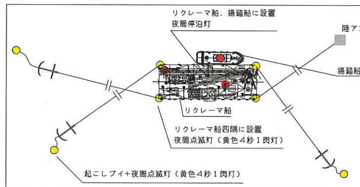
夜間停泊状況図
