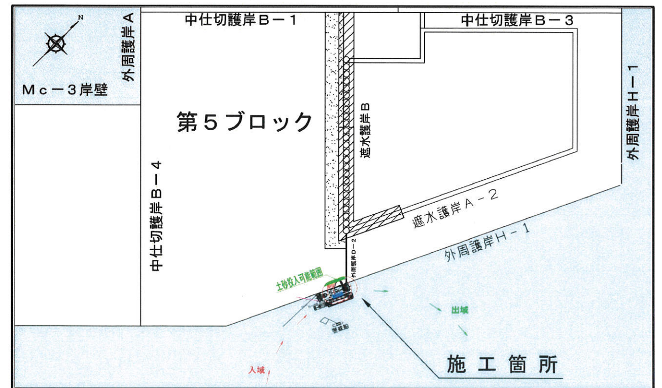
作業船配置図
