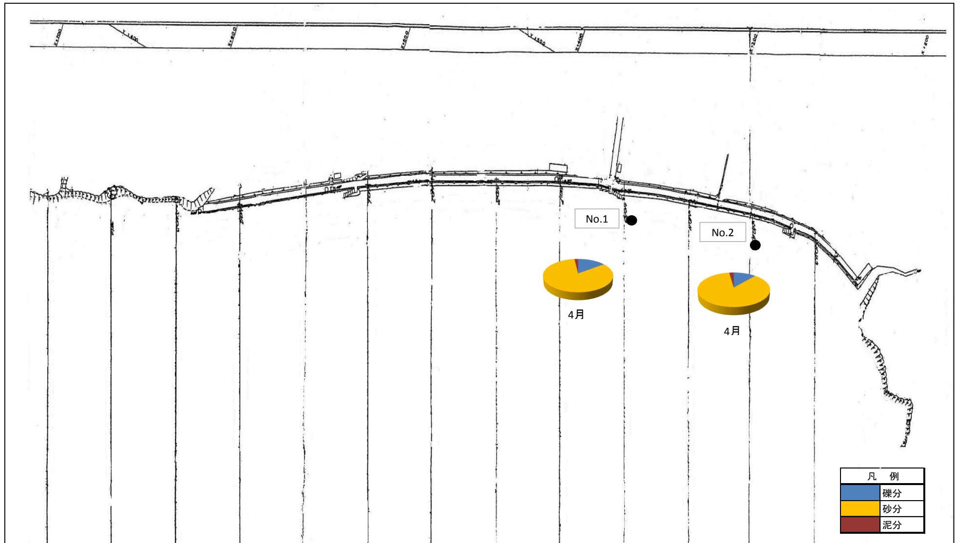
海老呑地区 粒度試験結果
